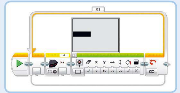
Рис. 14.13. Неполная программа для практикума № 74
