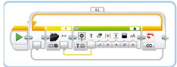
Рис. 14.17. Программа DisplayNumeric
