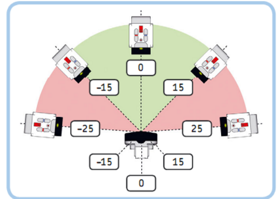
Рис. 8.8. Диапазон допустимых значений в режиме Направление маяка находится в пределах от -25 до 25. Отрицательные значения указывают, что маяк слева от датчика; положительные — что он справа. Значение, близкое к нулю, говорит о том, что робот обнаружил маяк прямо впереди или прямо сзади.
