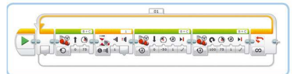
Рис. 6.6. Программа TouchAvoid. Блок Ожидание настроен на режим Датчик касания ▶ Сравнение ▶ Состояние
