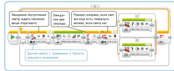
Рис. 7.17. Программа MazeCode. И первый блок Ожидание , и блок Переключатель находятся в режиме Датчик цвета -> Сравнение -> Яркость внешнего освещения
