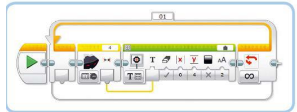
Рис. 14.17. Программа DisplayNumeric
